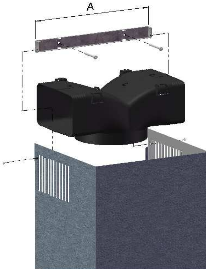
Abb. 1: Montageschema
