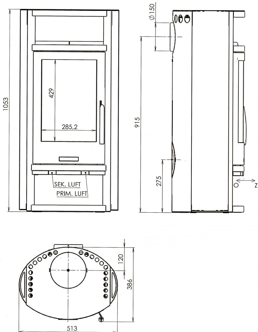
POLAR 4 - STAHL
